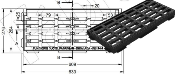
Grelha Sumidoura Anti-roubo C250 633x276x40 FAB.
